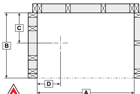
Vue de dessus de la structure
