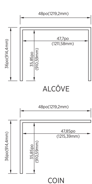
VUE DU DESSUS (ASSEMBLÉ)
